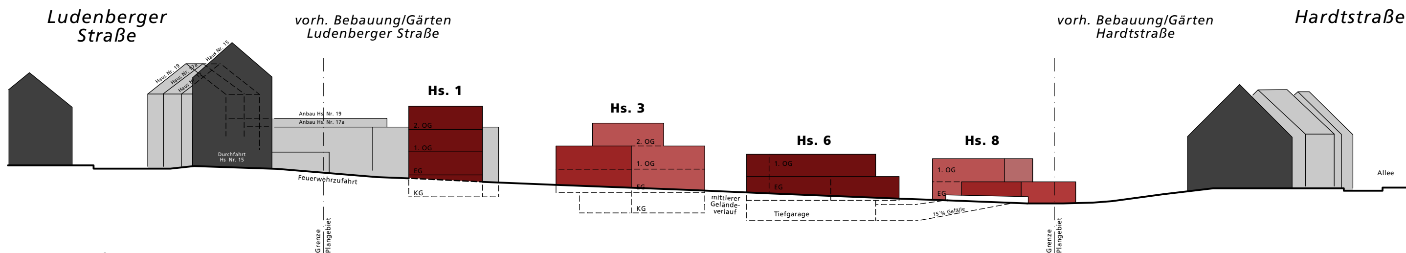
Längsschnitt A-A
